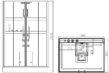
BẢN VẼ KÍCH THƯỚC
