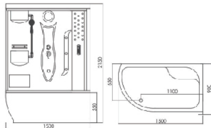
BẢN VẼ KÍCH THƯỚC
