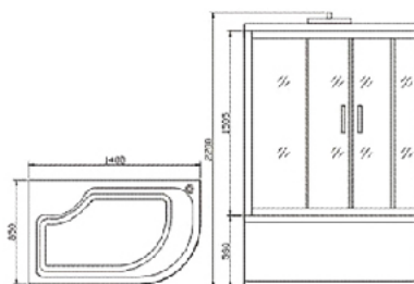
BẢN VẼ KÍCH THƯỚC
