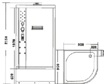
BẢN VẼ KÍCH THƯỚC
