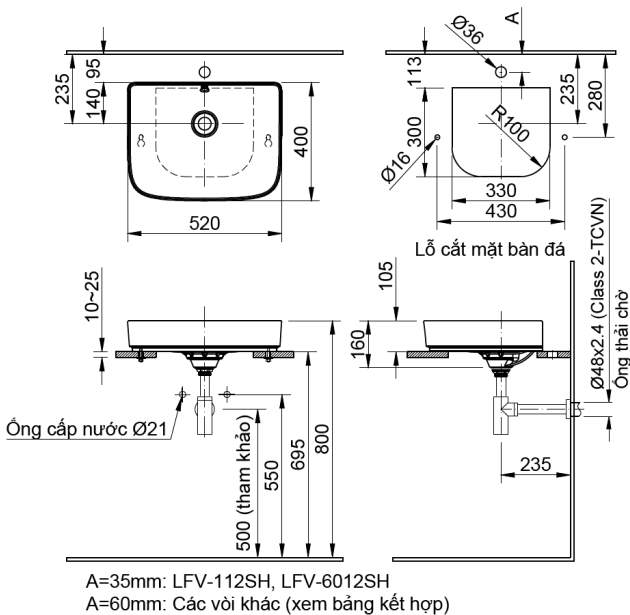
BẢN VẼ LẮP ĐẶT / INSTALLATION DRAWING
