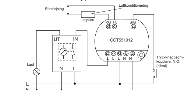
Fig 8. Sensorn används med en trappautomattimerkrets
