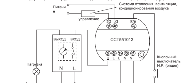
Рис. 8. Датчик, используемый с цепью лестничного таймера
