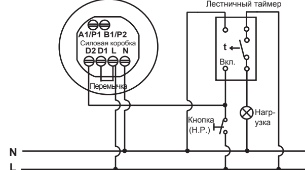
Рис. 5 3.2.1.2 Один датчик управляет системой отопления, вентиляции, кондиционирования воздуха (снимите проволочную перемычку на клеммах D1 и L).
