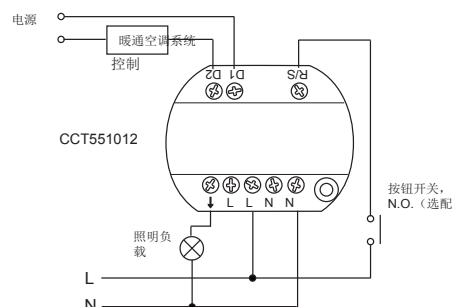
图 7. 典型双负载应用的接线图
