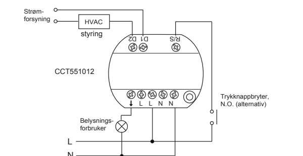
Fig 7. Koplingskjema for en typisk dobbeltlastbruk
