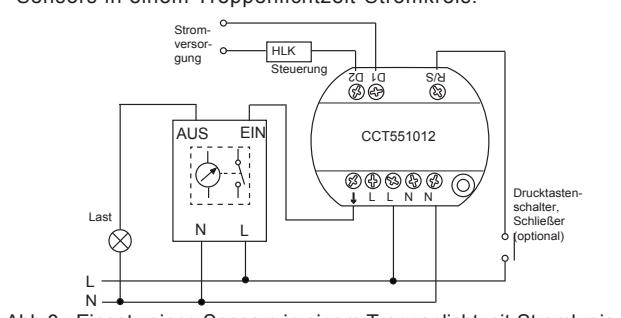
Abb 8. Einsatz eines Sensors in einem Treppenlichtzeit-Stromkreis
