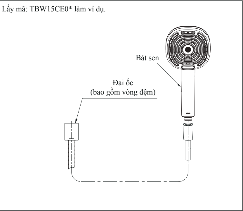
Hình 2: Lắp đặt dây sen với bát sen
